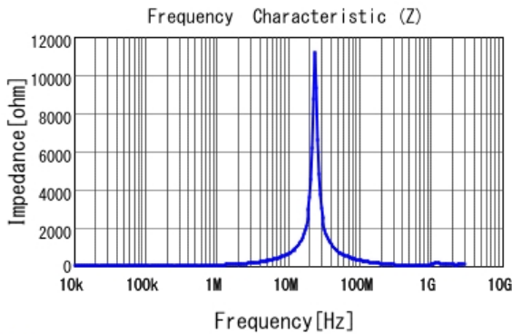
■ 1255AY-100M |Z|
