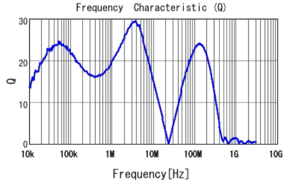
■ 1255AY-100M Q
