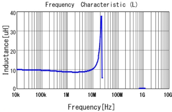
■ 1255AY-100M L
